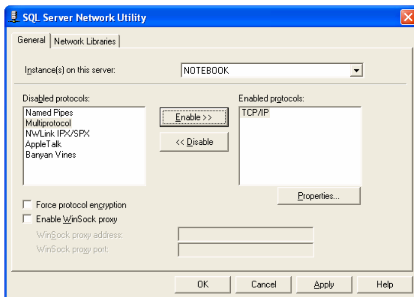
รูปที่ 5-28 รูปแสดงหน้าต่าง SQL Server Network Utility
