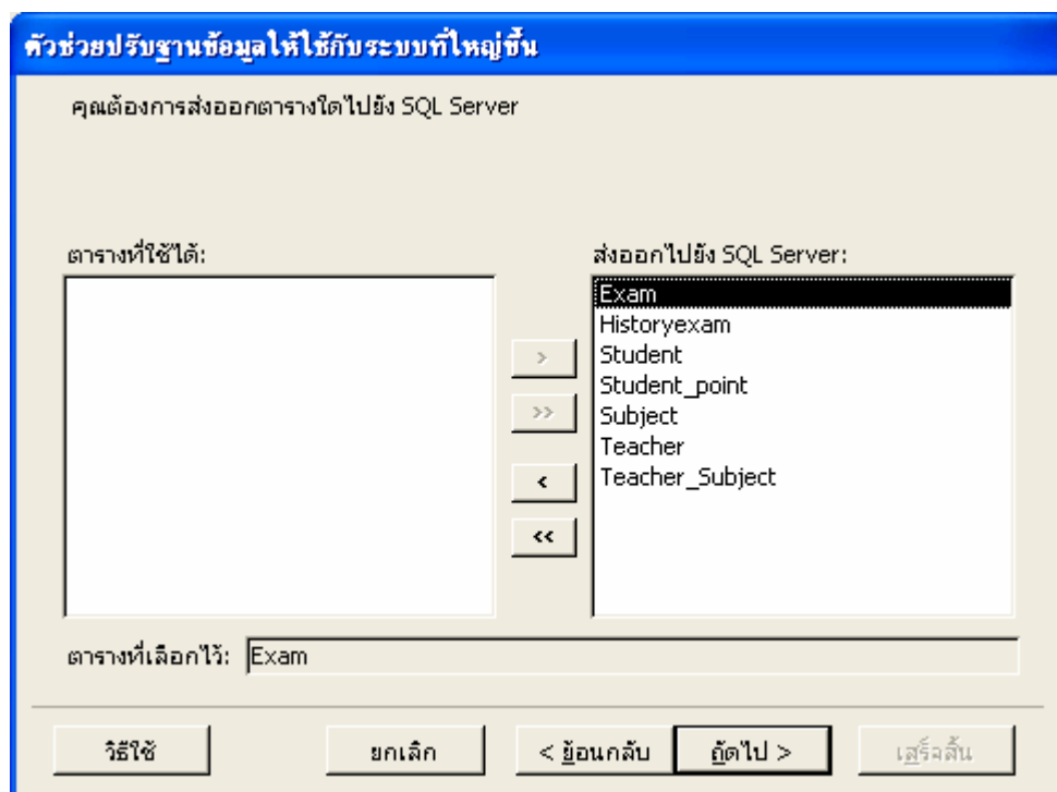
รูปที่ 5-32 รูปแสดงการเลือกตารางเพื่อนำมาใช้งานใน MSDE
