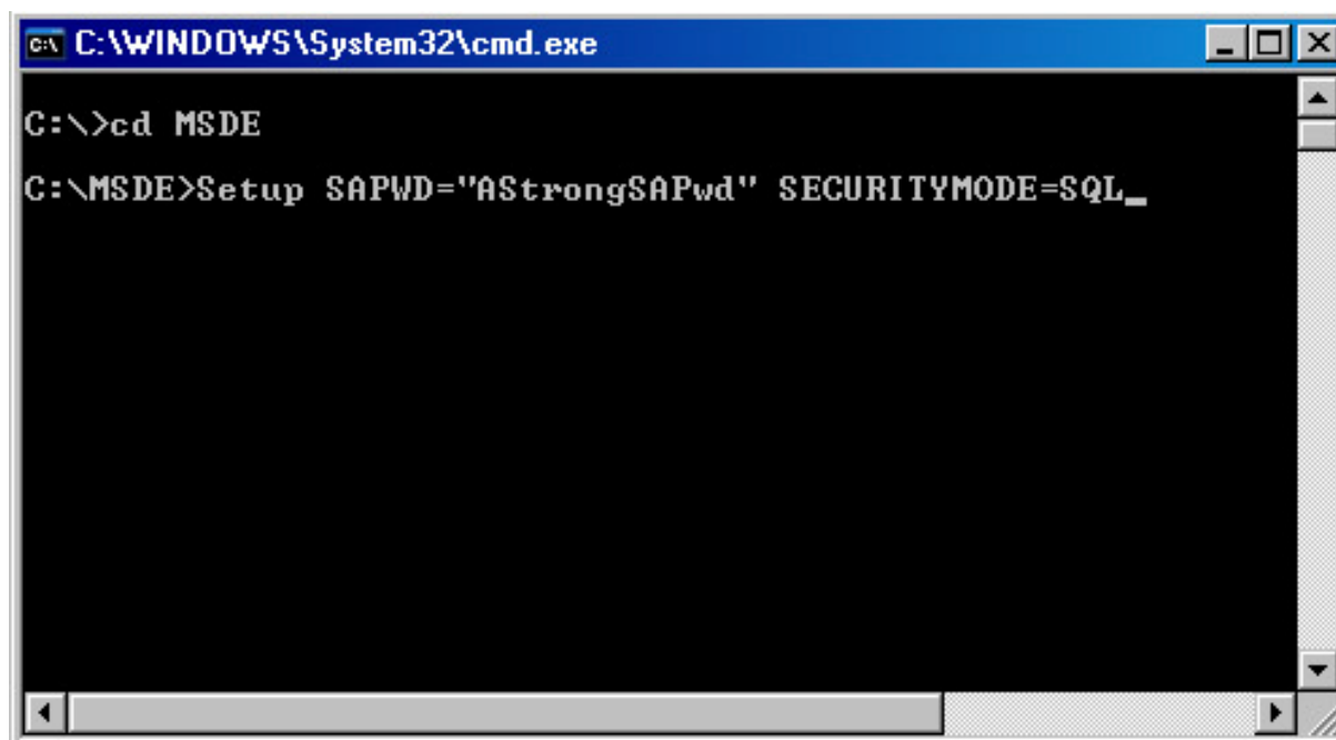
รูปที่ 5-27 รูปแสดงคำสั่งการติดตั้งโปรแกรม MSDE
